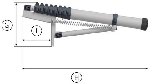
Loft Line yttermått
